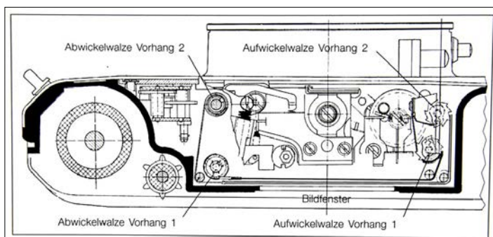
Tegning af spaltelukkeren set fra bunden af kameraet.
